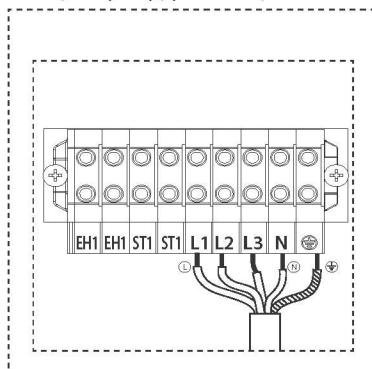
Κιβώτιο διασύνδεσης εξωτερικής μονάδας 3Ph
