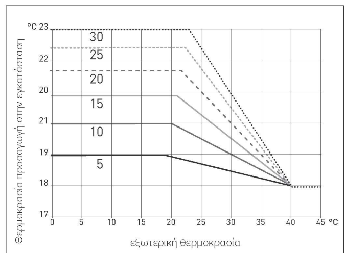
Γράφημα Β (εγκατάσταση σε δάπεδο)
