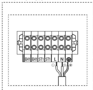
Κιβώτιο διασύνδεσης εξωτερικής μονάδας 1Ph
