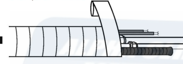
Βήμα 7: Τυλίξτε με ταινία τον σωλήνα και το καλώδιο
